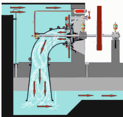
Princip průtoku vody Francisovou turbínou
